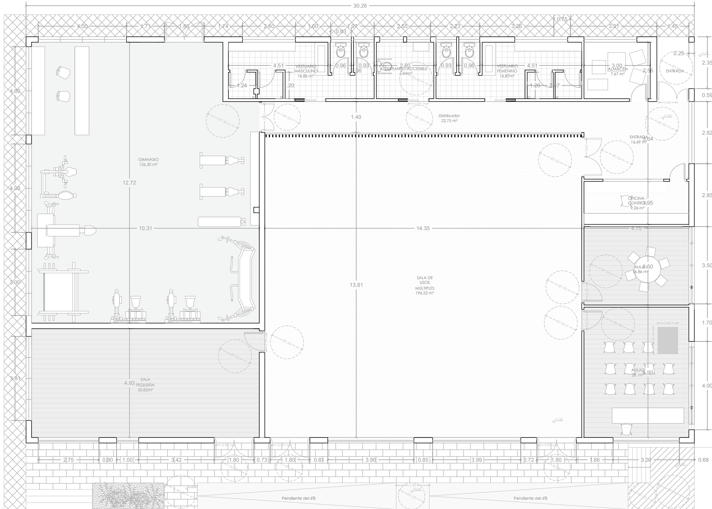
Planta Baja +4.50 m
